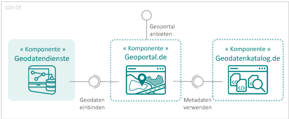
Abbildung 13: Komponentendiagramm Geoportal.de
